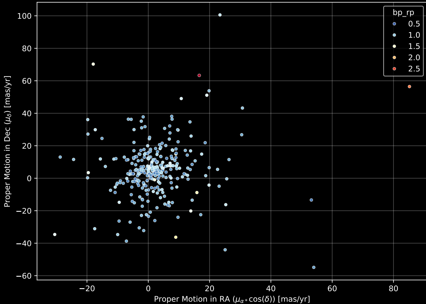
GALAH DR4 Field: [658] Proper Motion Diagram (n= 294)
